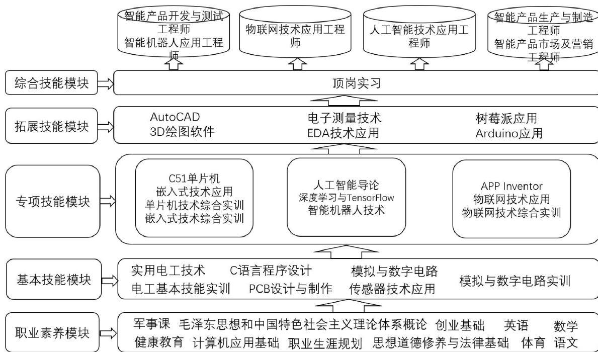
图 1 课程体系图
